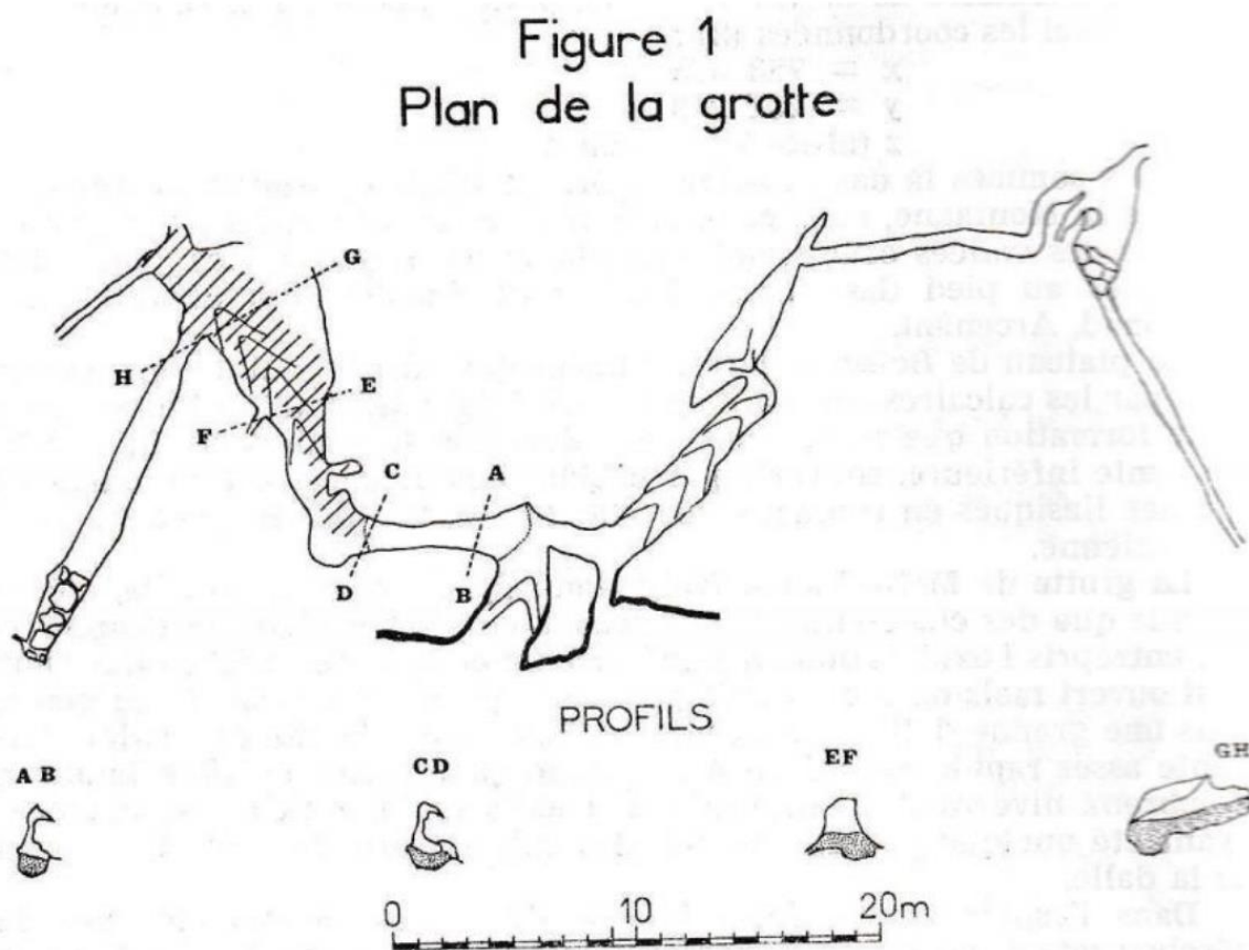
FIGURE 1 Plan de la grotte de Molle Pierre
